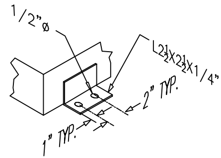
FOOT DETAIL SCALE: N.T.S.
